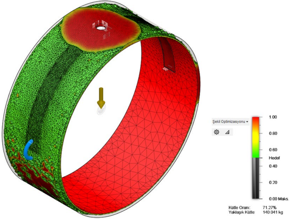
Şekil 2. Strateji 1'e göre elde edilen topoloji optimizasyon sonucu: malzeme dağılımı deformasyonu minimize edecek şekilde düzenlenmiştir.
