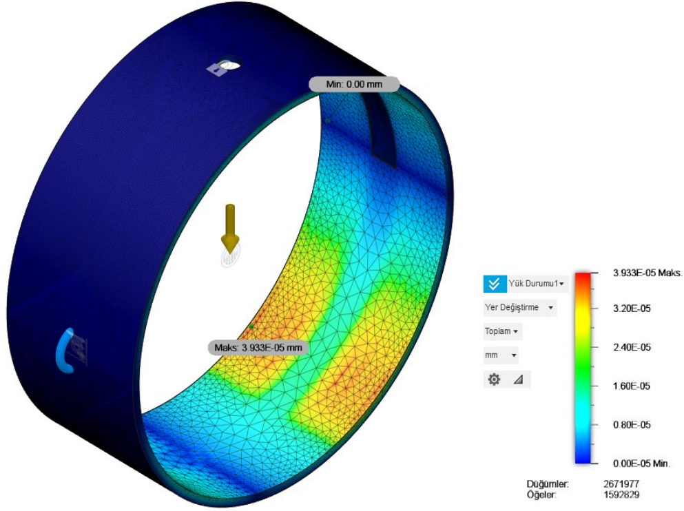
Şekil 6. Optimize edilmiş modelin yer değiştirme (deformasyon) grafiği.
