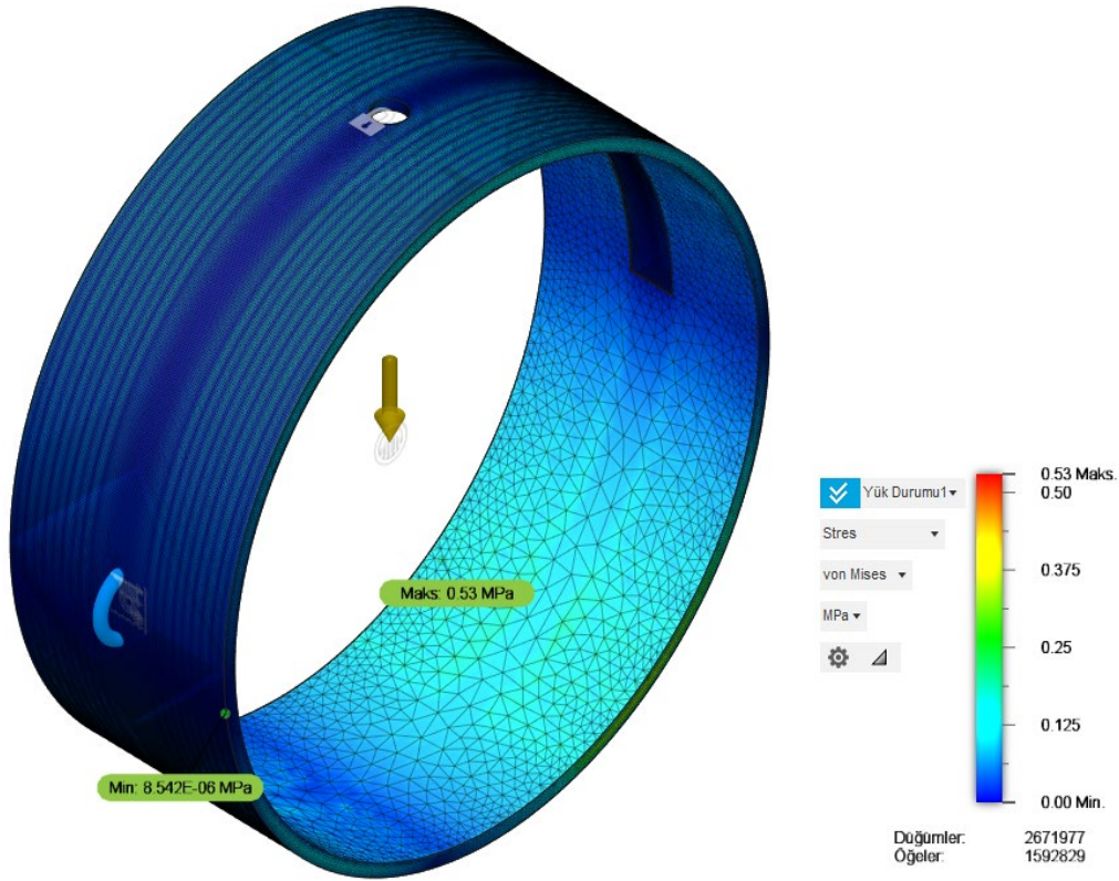
Şekil 5. Topoloji optimizasyonuna göre revize edilen modelin statik analiz gerilme sonuçları.
