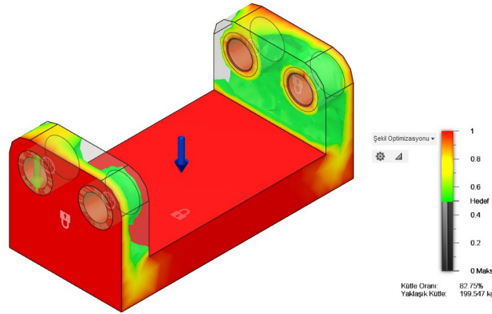
Şekil 1. Fusion 360 ortamında gerçekleştirilen topoloji optimizasyonu işlemine ait örnek görüntü, malzeme azaltımı yapılan bölgeler belirgin şekilde görünmektedir.
