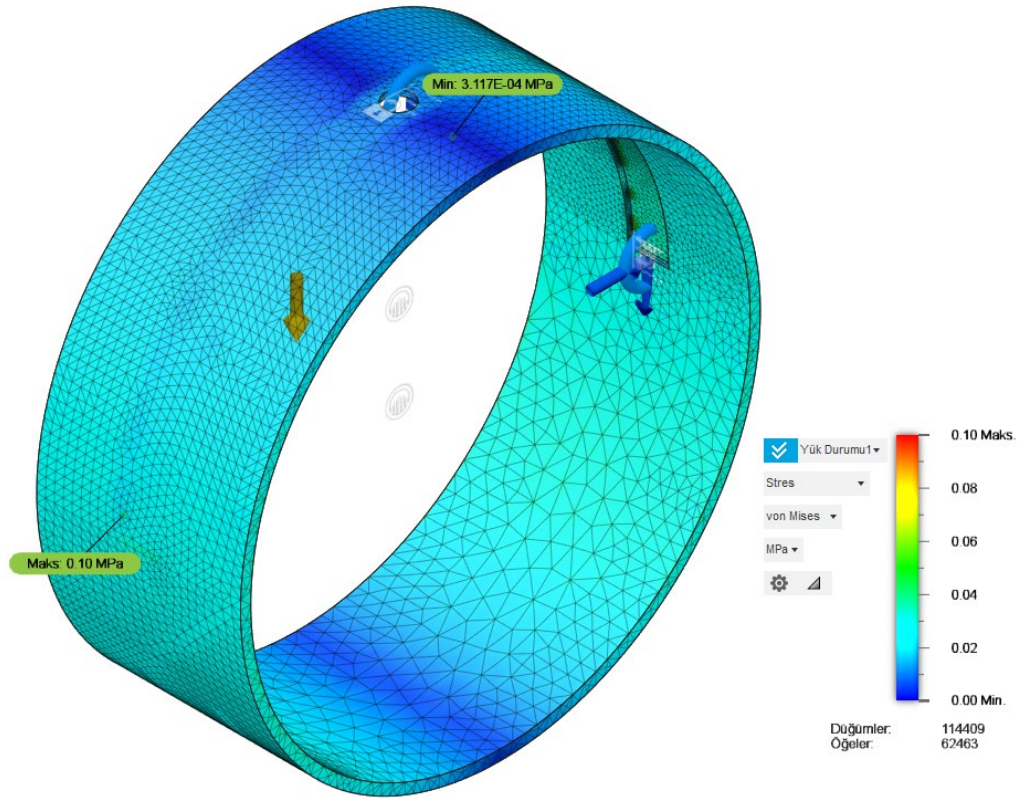
Şekil 3. En uygun üretken tasarım modeline ait statik analiz sonuçları.
