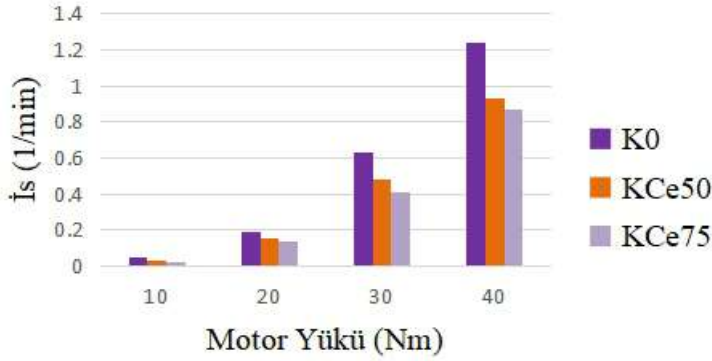
Şekil 6. Dizel yakıtı içerisinde ilave edilen NPs is emisyonlarına etkisi etkisi (Çelik & Bayındırlı, 2024a)
